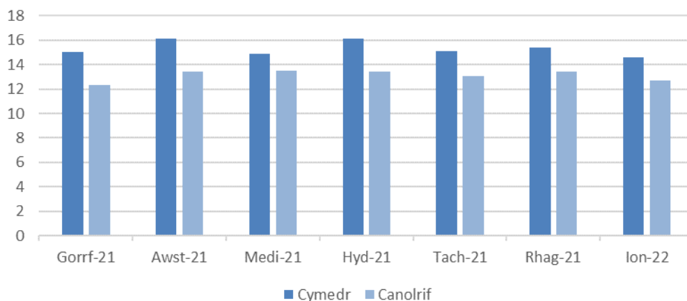
Ffigur 3.2: Hyd cyfveliadau ar-lein ar gyfartaledd yn ôl mis yr arolwg mewn munudau
