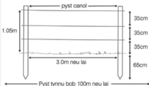
Diagram o Ffens Weiren Tri Llinyn
